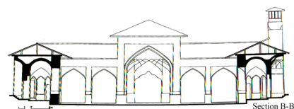
تصویر ۱۴. پلان و مقطع مسجد جامع بابل. مأخذ: پرونده ثبتی، اداره کل میراث فرهنگی، گردشگری و صنایع دستی استان مازندران.
